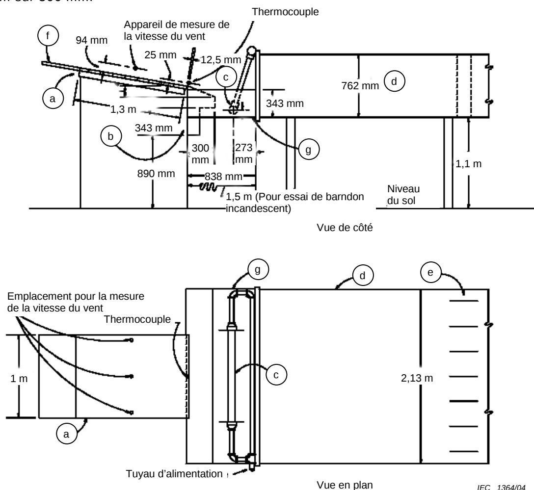
Figure A.1 – Appareillage d'essai pour l'essai d'inflammabilité http://solargostaran.com
